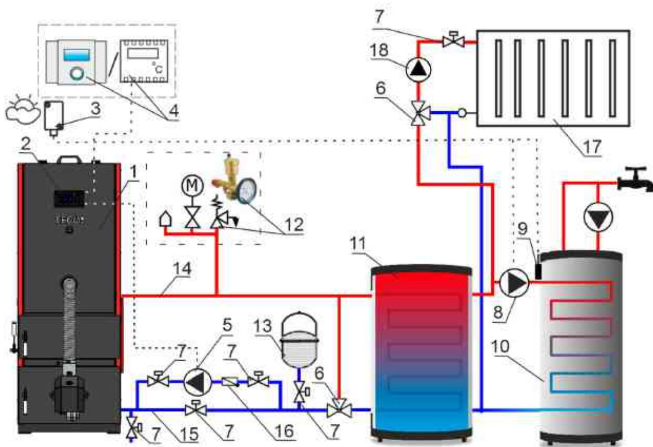
Рис. 14 Гидравлическая схема подключения 1
